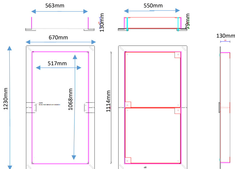
Jesmig Teknik 563x1114 m/2 dæksler
