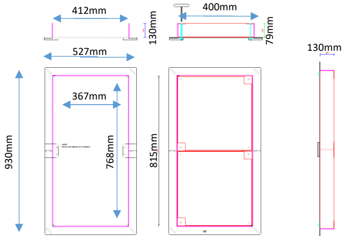
Jesmig Teknik 412x815 m/2 dæksler
